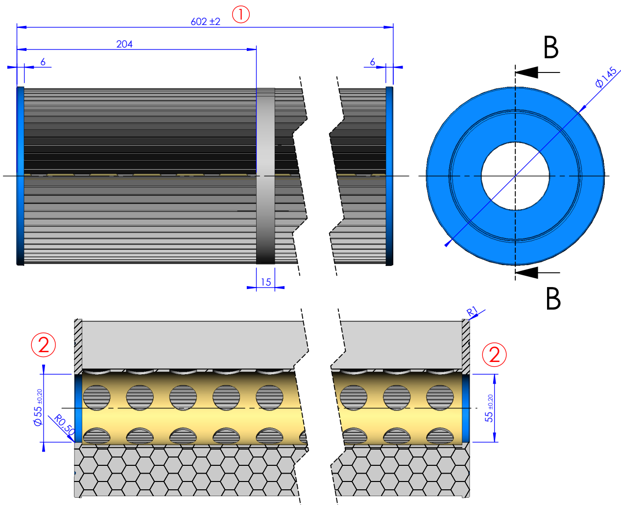
Secció B-B
